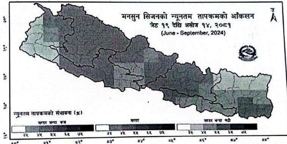
चित्र ३: २०८१ को मनसुन सिजनको न्यूनतम तापक्रम (सरदर भन्दा कम वा सरदर वा सरदर भन्दा बढी) को सर्वाधिक सम्भावना (highest probability) (%)
