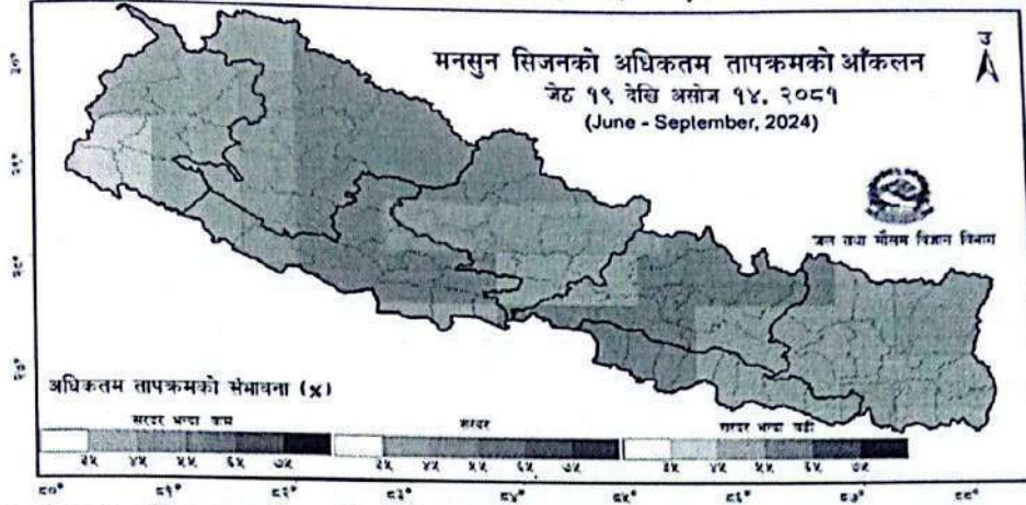
चित्र २: २०८१ को मनसुन सिजनको अधिकतम तापक्रम (सरदर भन्दा कम वा सरदर वा सरदर भन्दा बढी) को सर्वाधिक सम्भावना (highest probability) (%)
